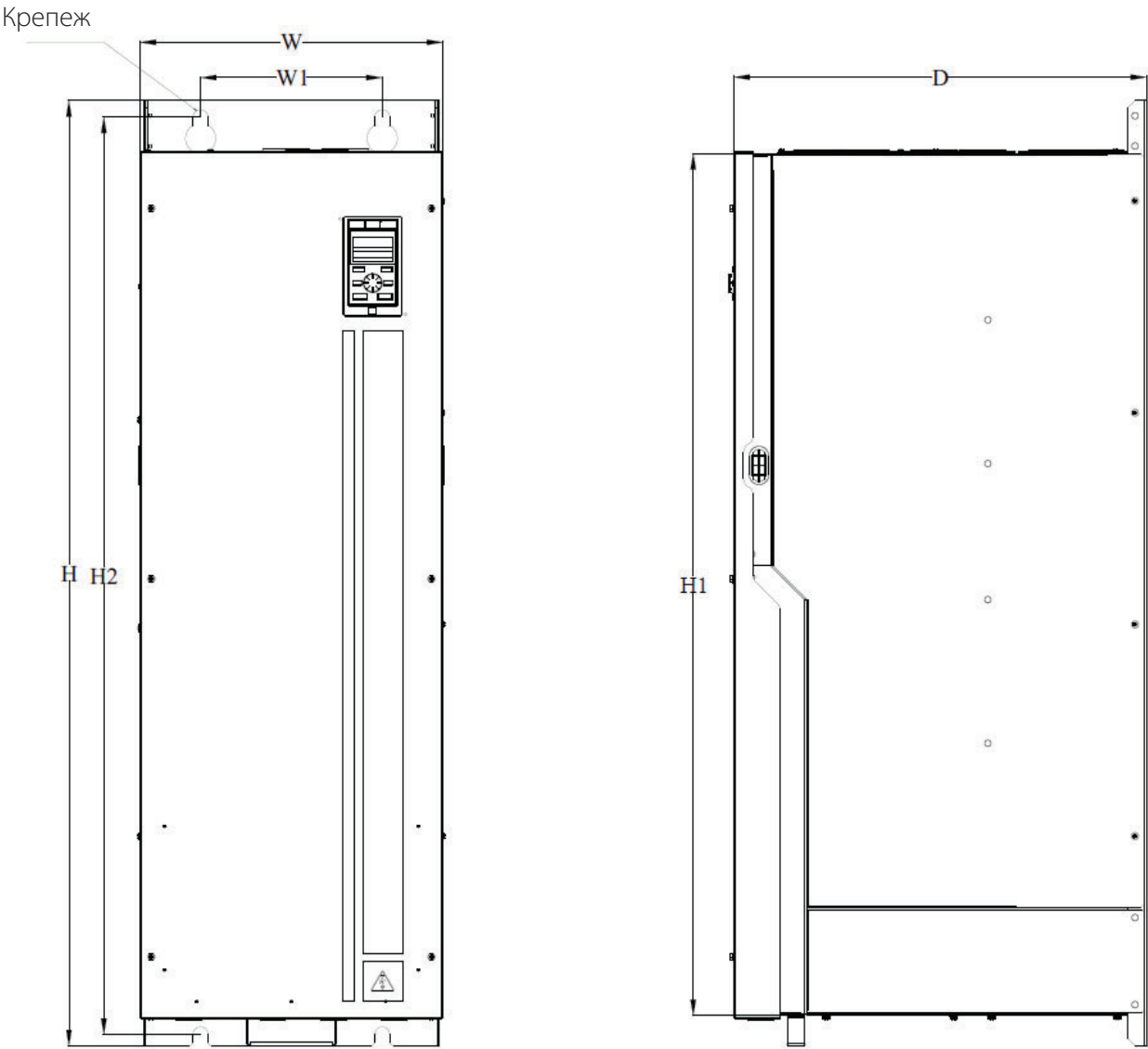
Рис.2-6.10. Чертеж преобразователя частоты типоразмер В10
