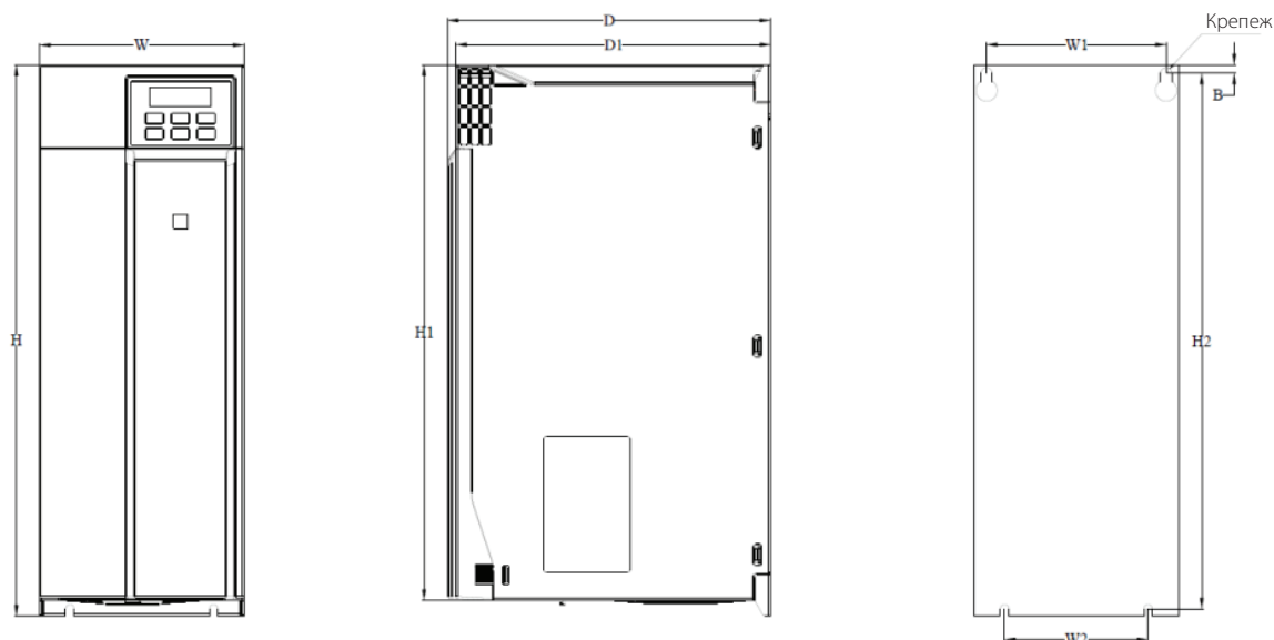
Рис.2-6.4. Чертеж преобразователя частоты типоразмер В4
