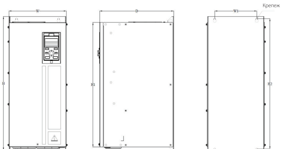
Рис.2-6.6. Чертеж преобразователя частоты типоразмер B6
