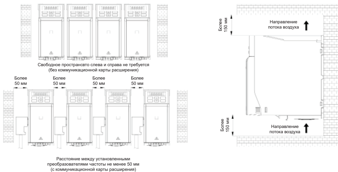
Рис. 2-5 Положение преобразователя частоты и требуемое пространство
