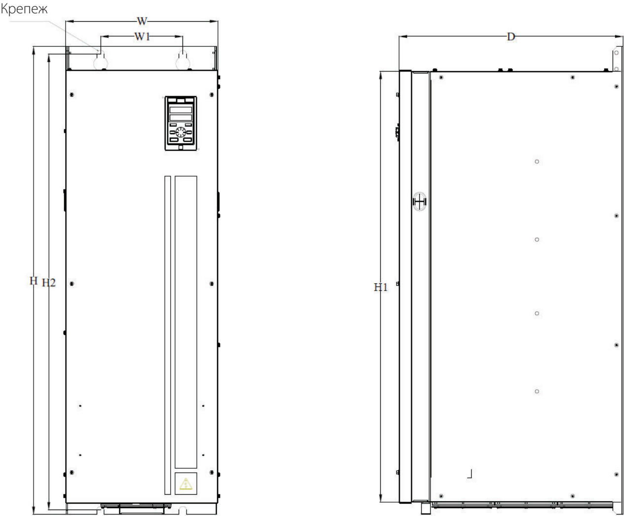
Рис.2-6.9. Чертеж преобразователя частоты типоразмер В9 Таблица 2-6.9 Габаритные размеры преобразователя частоты типоразмер В9
