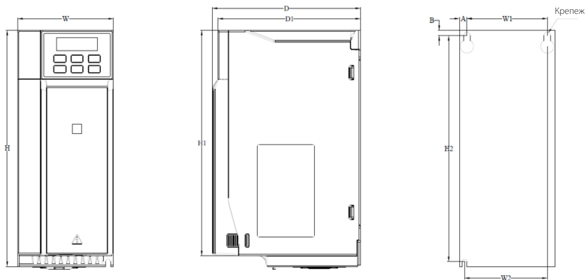
Рис.2-6.2. Чертеж преобразователя частоты типоразмер В2
