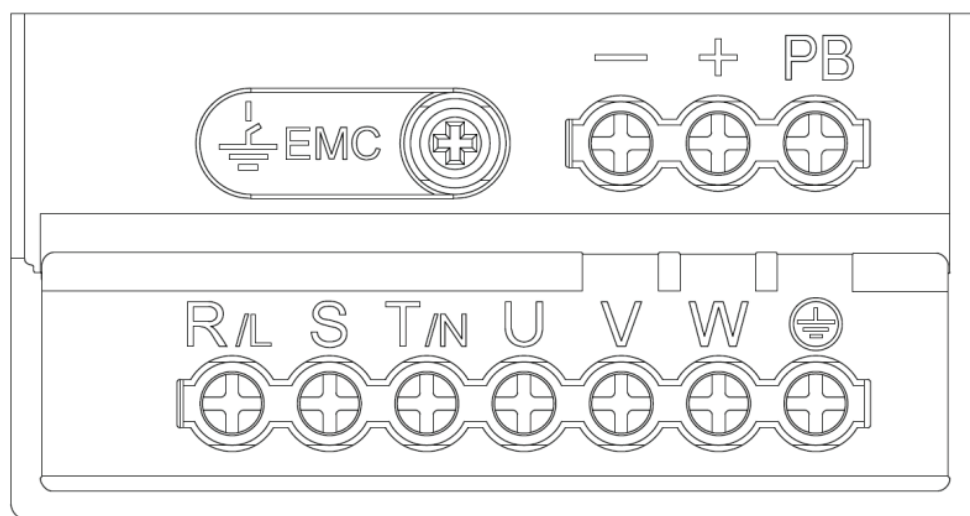
Рис. 3-3.2 Расположение клемм
