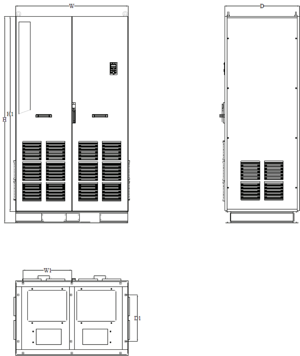
Рис.2-6.12. Чертеж преобразователя частоты типоразмер В12
