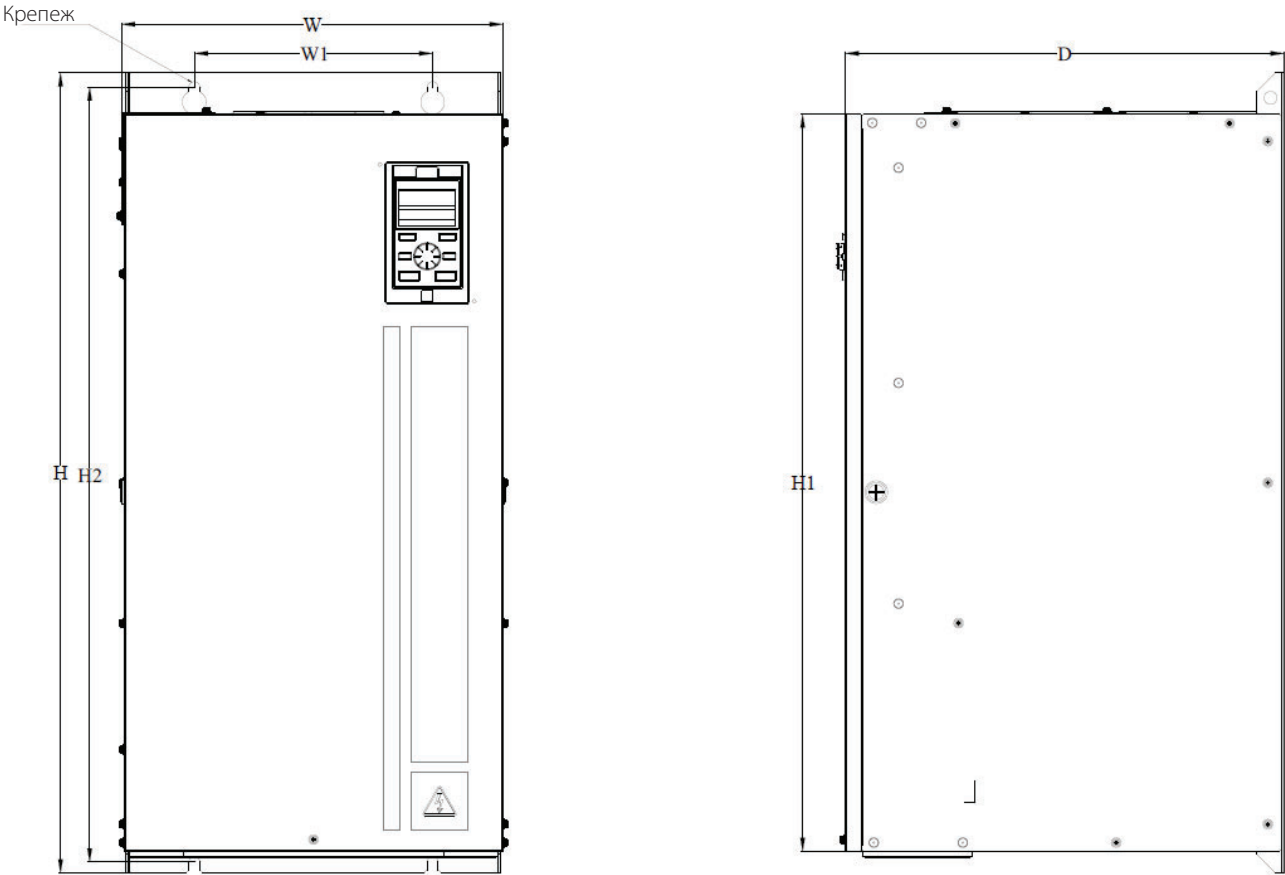
Рис.2-6.7. Чертеж преобразователя частоты типоразмер В7
