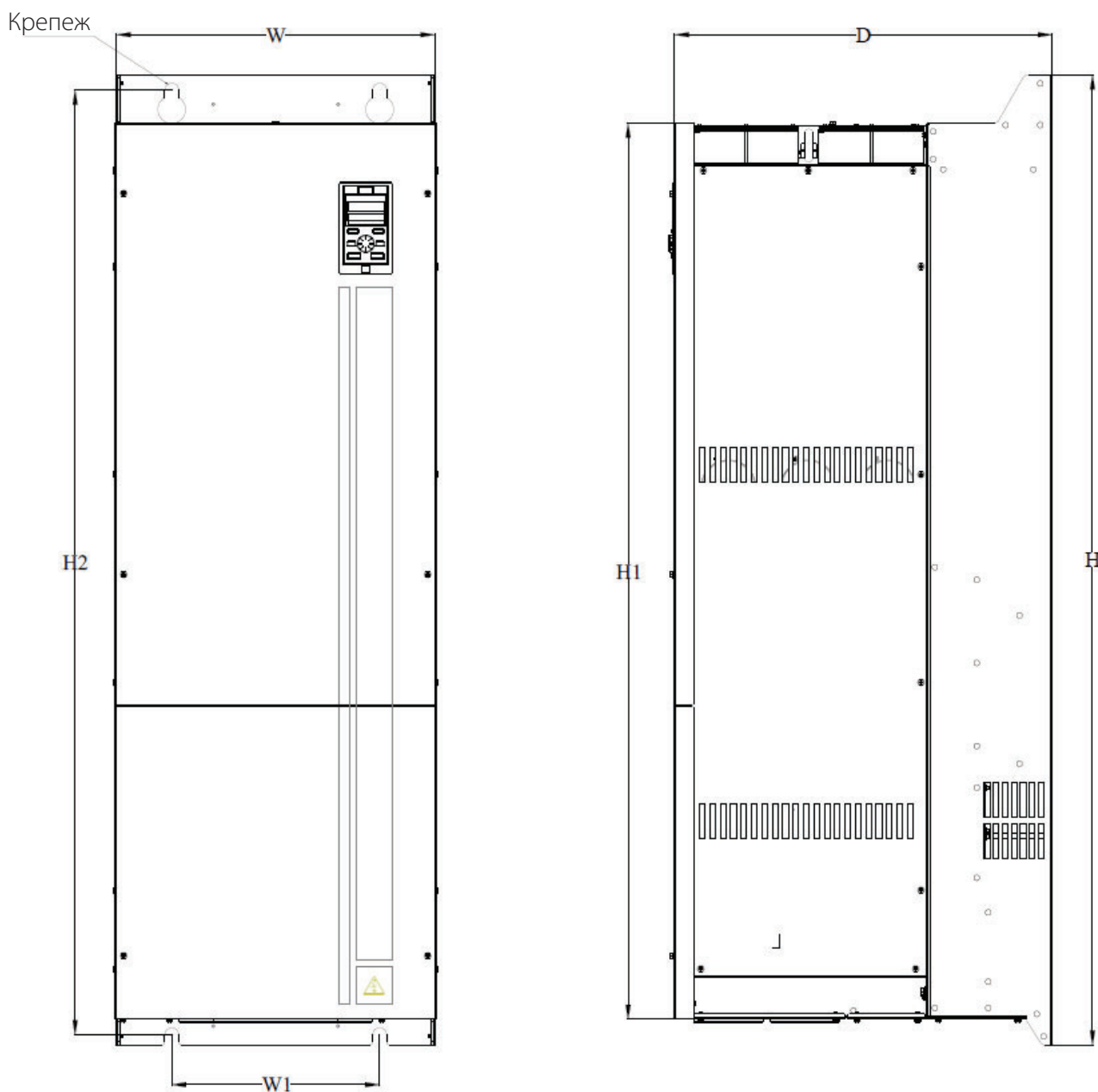
Рис.2-6.11. Чертеж преобразователя частоты типоразмер В11
