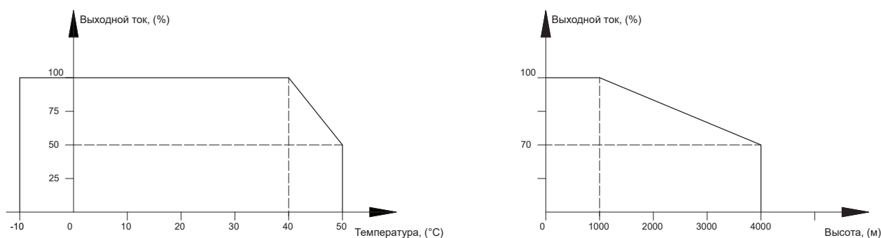
Рис. 2-4 Снижение характеристик преобразователя частоты при превышении допустимой температуры и высоты
