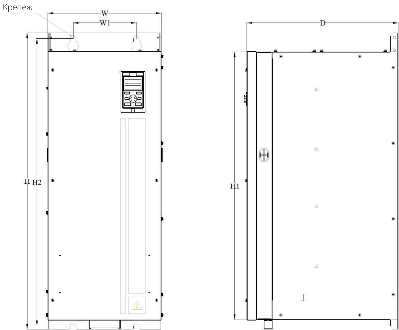
Рис.2-6.8. Чертеж преобразователя частоты типоразмер В8
