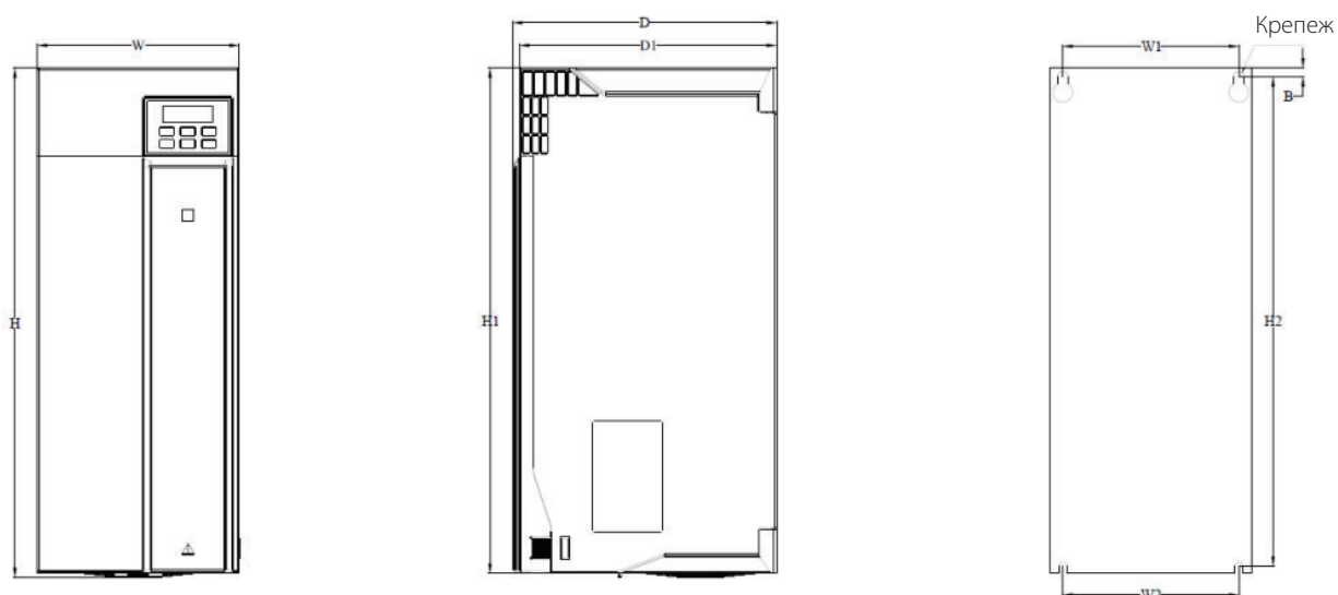
Рис.2-6.5. Чертеж преобразователя частоты типоразмер B5
