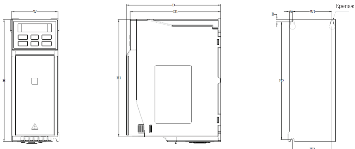
Рис.2-6.1. Чертеж преобразователя частоты типоразмер В1
