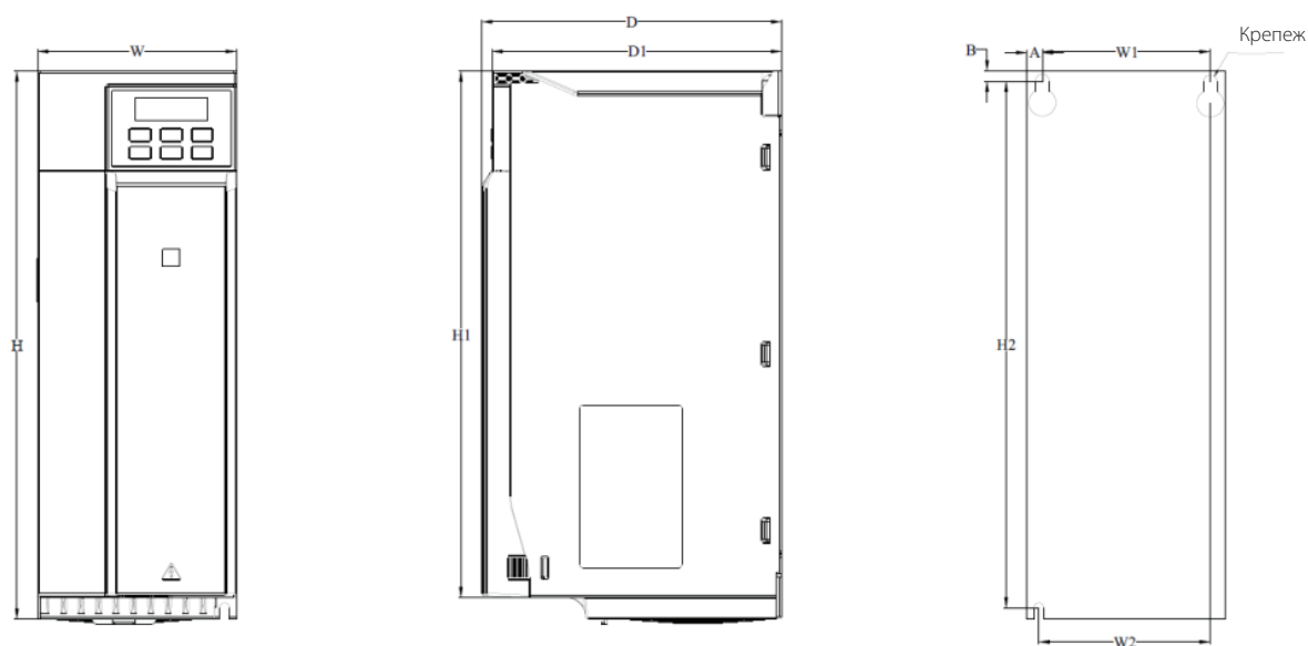
Рис.2-6.3. Чертеж преобразователя частоты типоразмер В3
